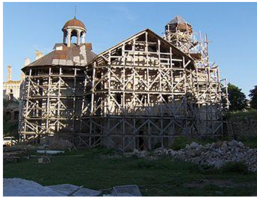
Рис. 3.1 – Реставраційне риштування Бережанського замку
